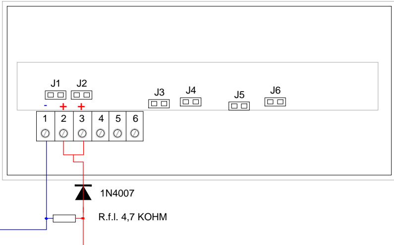
OPTICAL ACUSTIC DISPLAY - TARGA OTTICO ACUSTICA - mod. FD5955
